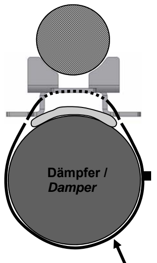
Dämpfer / Damper Kabelbinder / Cable ties
