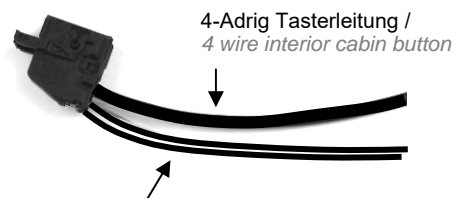
Klemme 15 und Geschwindigkeit / Clamp 15 and speed
